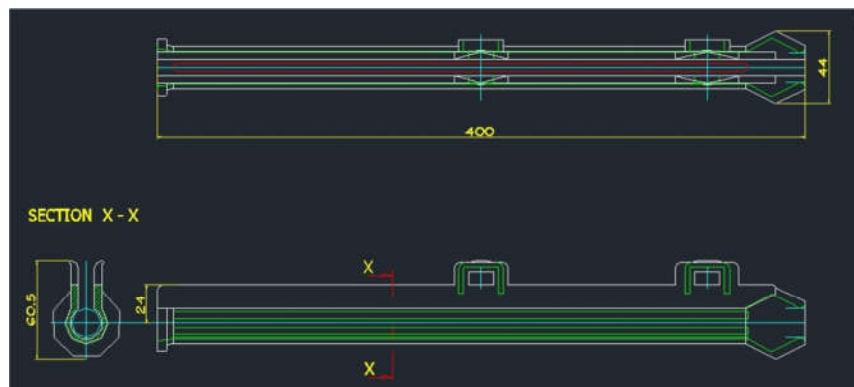
DIMENSI TEKEP ISOLATOR EXTENTION
